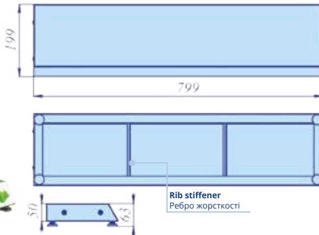
Р3.093-01 Metall stand Підставка з металу
