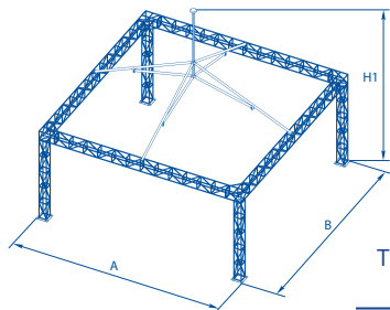
PAVILION DOMICAL, REINFORCED ПАВІЛЬЙОН КУПОЛЬНИЙ, ПОСИЛЕНИЙ
