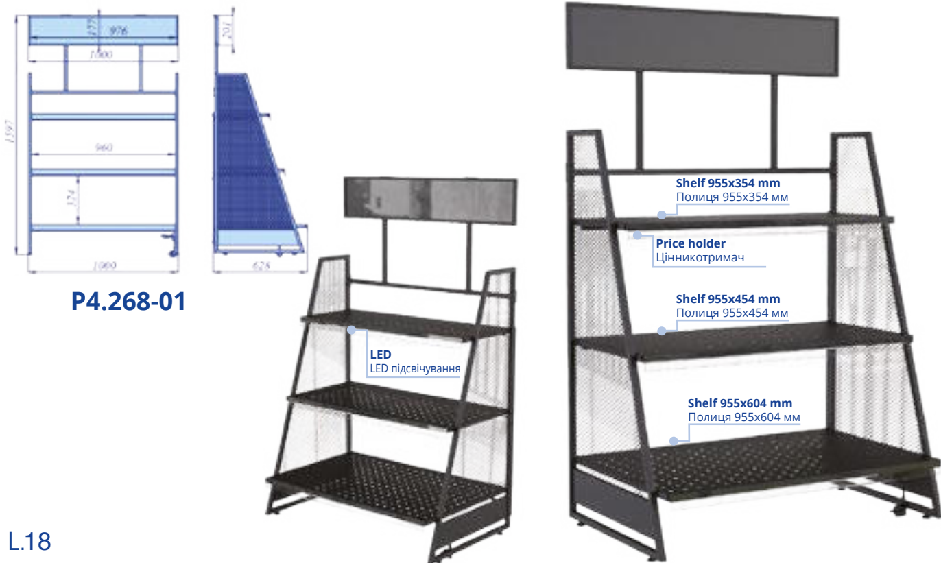
Illuminated rack Стелаж з підсвічуванням
