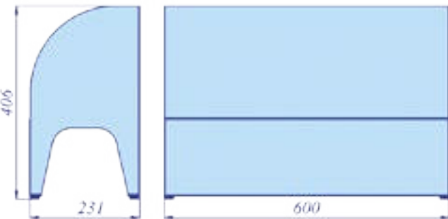
Р3.163-01 Metall stand Підставка з металу
