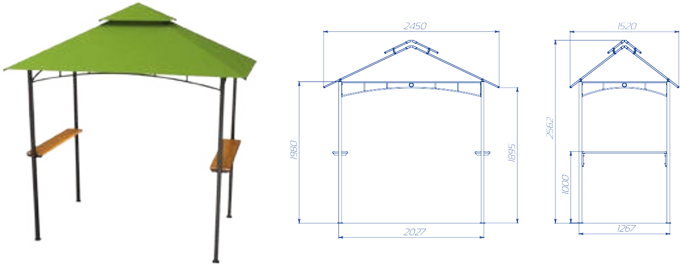
HOLIDAY TENT 3X3 НАМЕТ ДЛЯ ВІДПОЧИНКУ 3Х3
