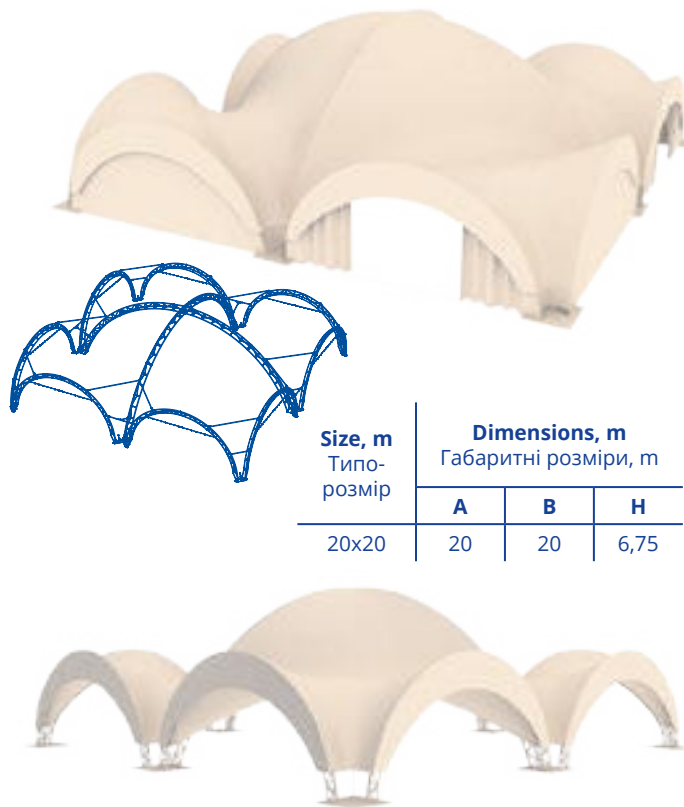
20x20 PAVILION ПАВІЛЬЙОН «20x20»
