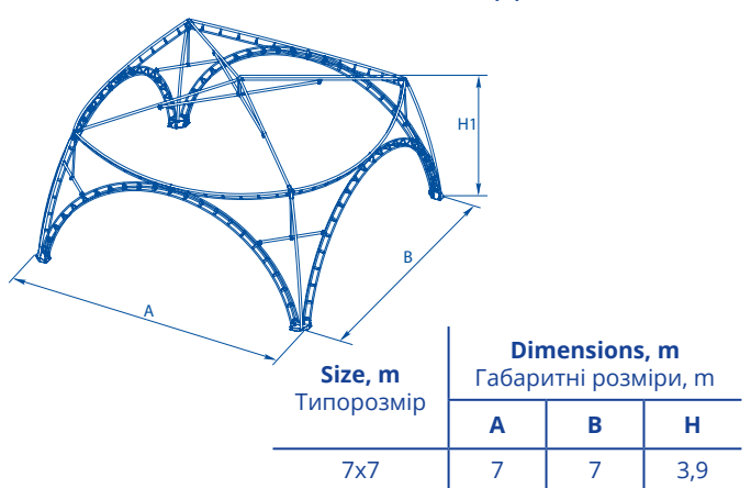
NON-STANDARD PAVILION ПАВІЛЬЙОН НЕСТАНДАРТНИЙ
